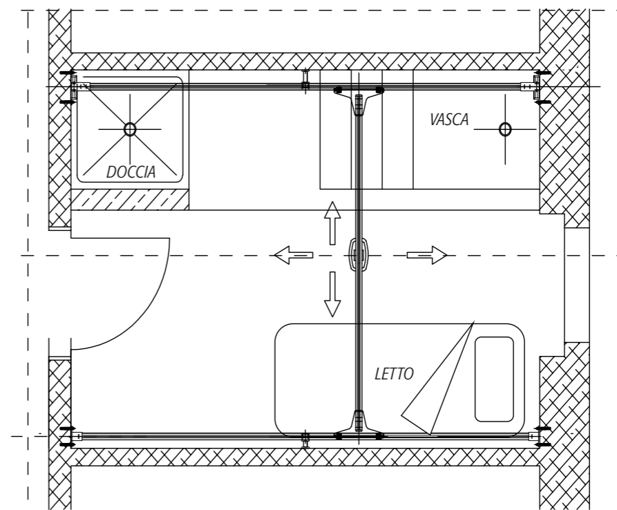
Movimentazione a "binario" Ceiling "Track" system
